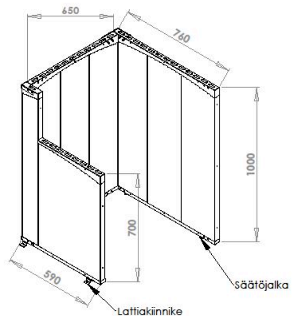
Tulisijan suojaseinän asennuskuvat
